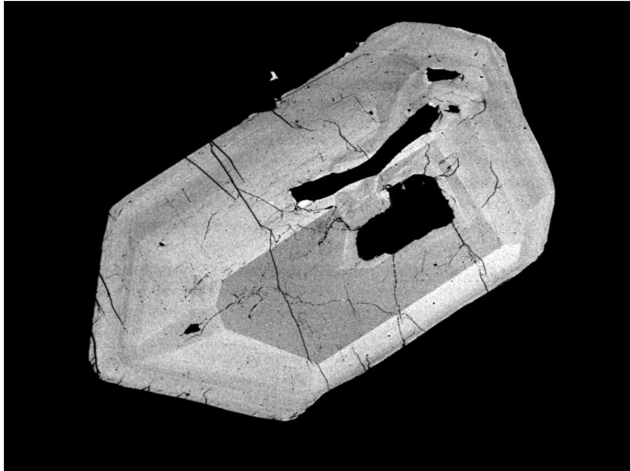
Mineral: Monazite
