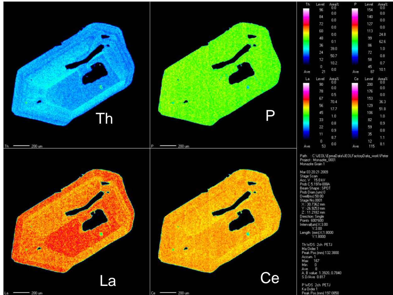
Mineral: Monazite
